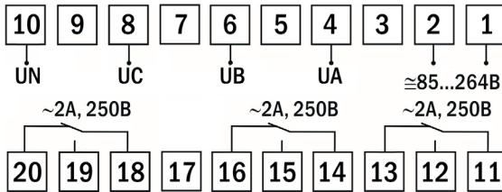
Рис. 4 – Схема подключения
