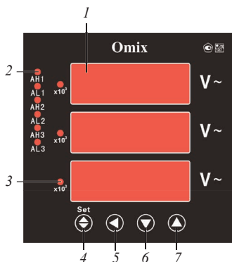
Рис. 1 – Управляющие элементы
