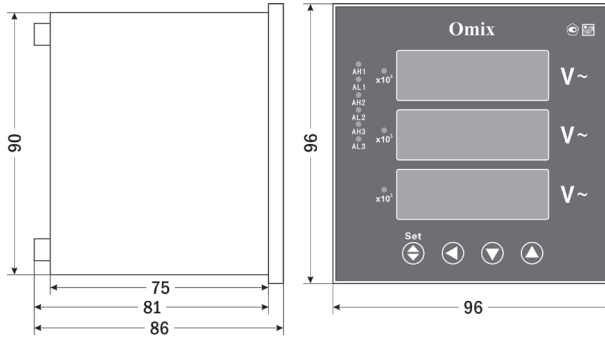
Рис. 3 – Размеры прибора
